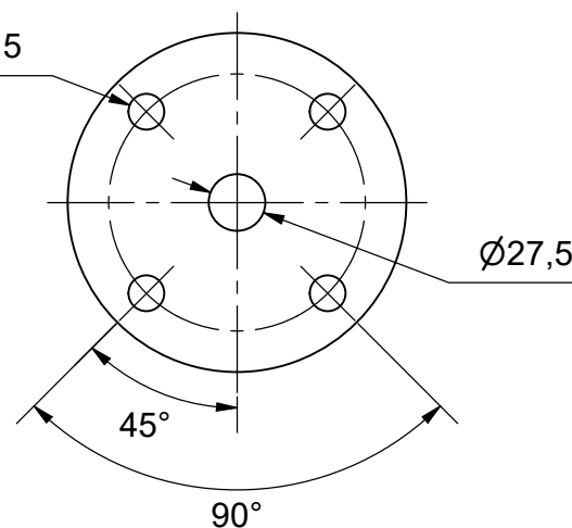
Sheet Plate ( 1 : 4 )
